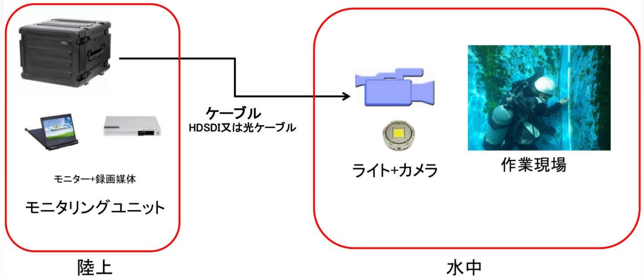
seatoolの陸上モニタリングシステム
